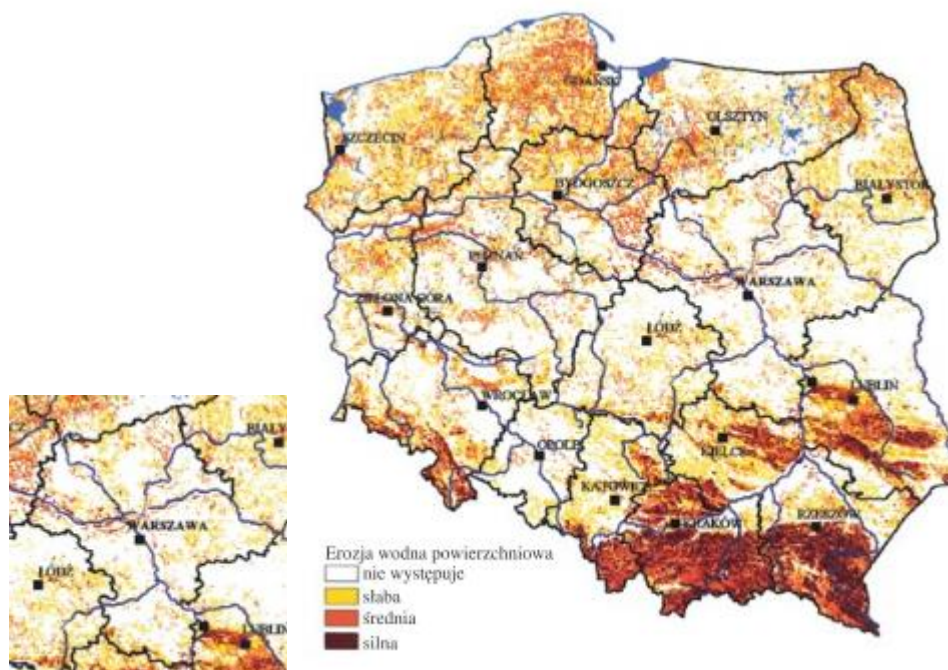
Rysunek 11. Mapa potencjalnej erozji wodnej
