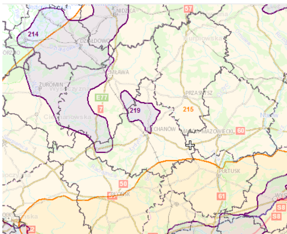
Rysunek 5. Główne zbiorniki wód podziemnych na terenie powiatu ciechanowskiego 33
