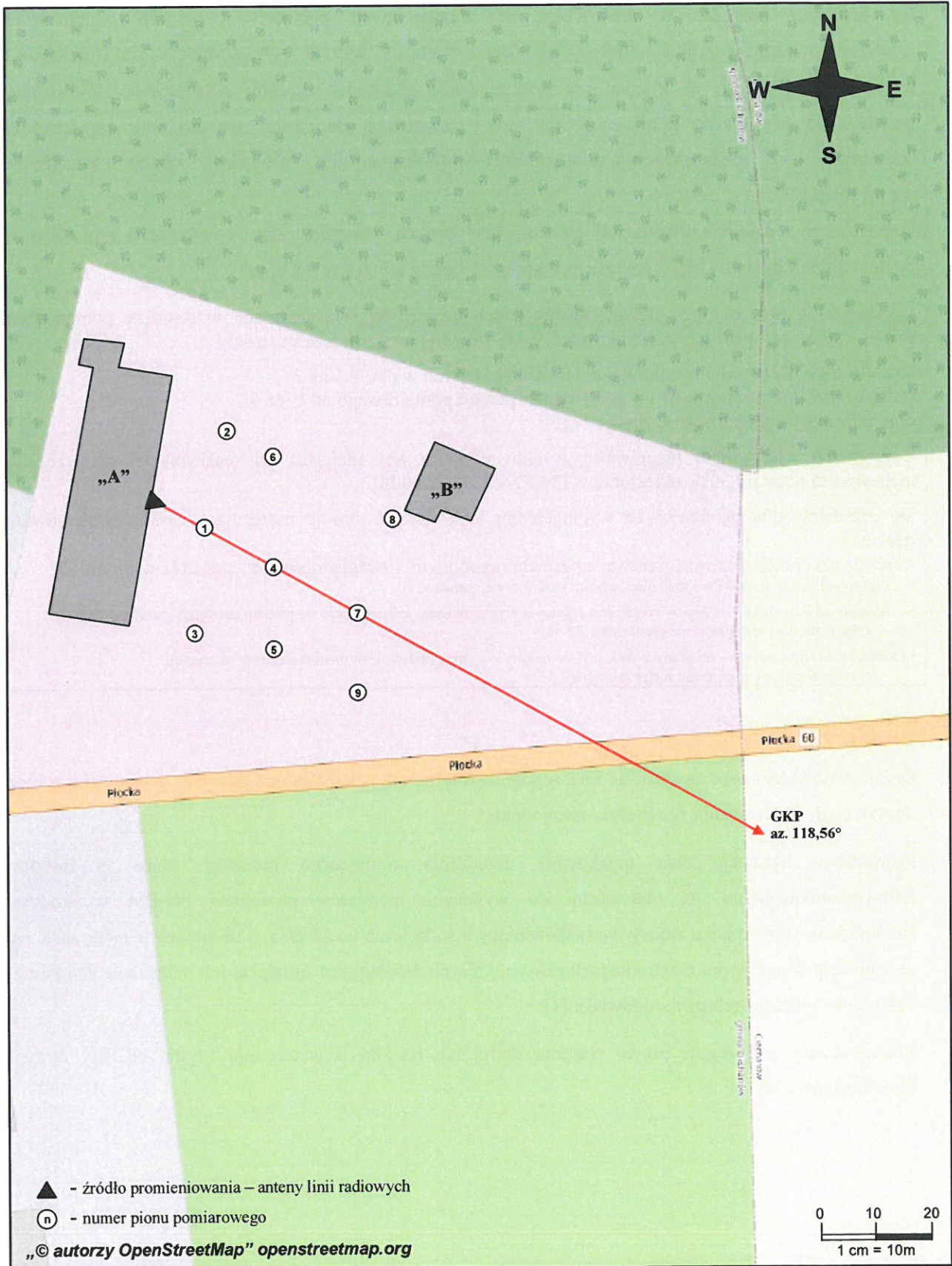
Rys. 1. Usytuowanie punktów i pionów pomiarowych w otoczeniu instalacji radiokomunikacyjnej Stacja Netia CIEWB085-CIEWM00020 Pęczcin, ul. Płocka 2
