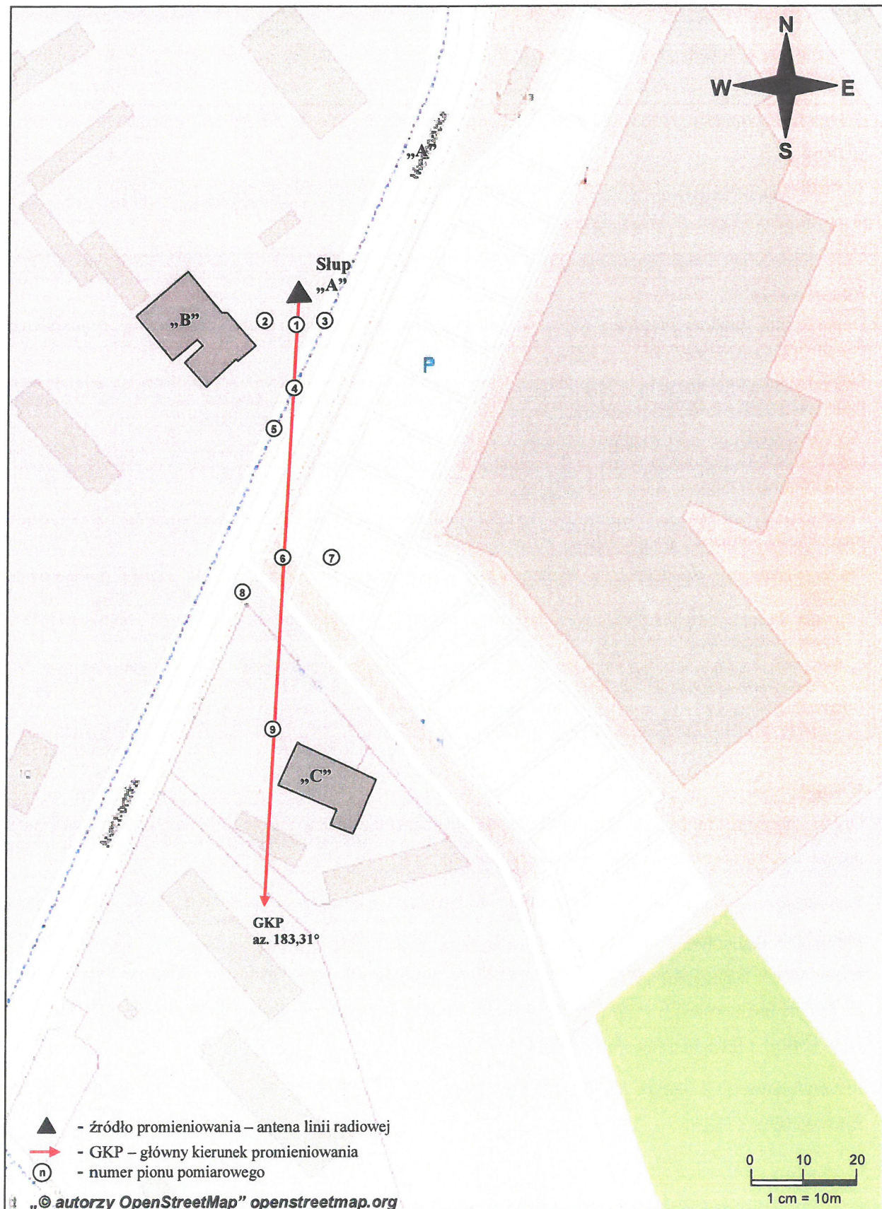
Rys. 1. Usytuowanie punktów i pionów pomiarowych w otoczeniu instalacji radiokomunikacyjnej Stacja Netia CIEWB079-CIEWM00018 Ciechanów, ul. Niechodzka 6
